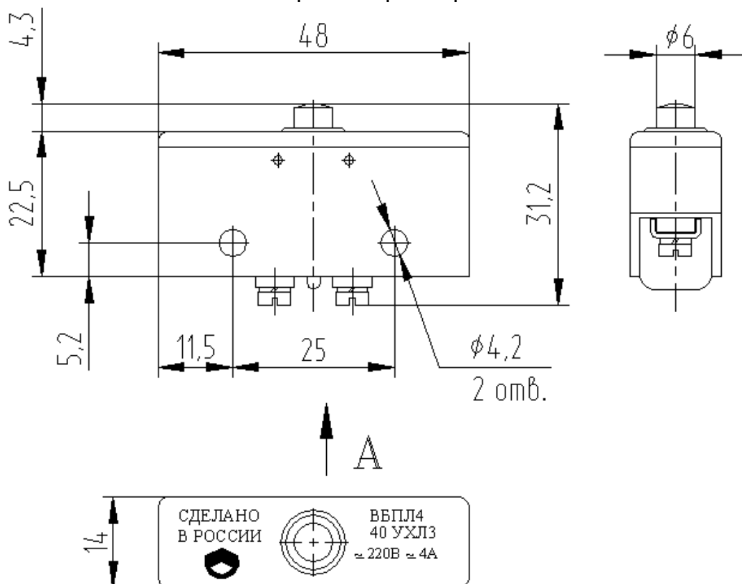
Габаритные размеры
